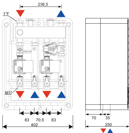
T-BOX 2x DN20
